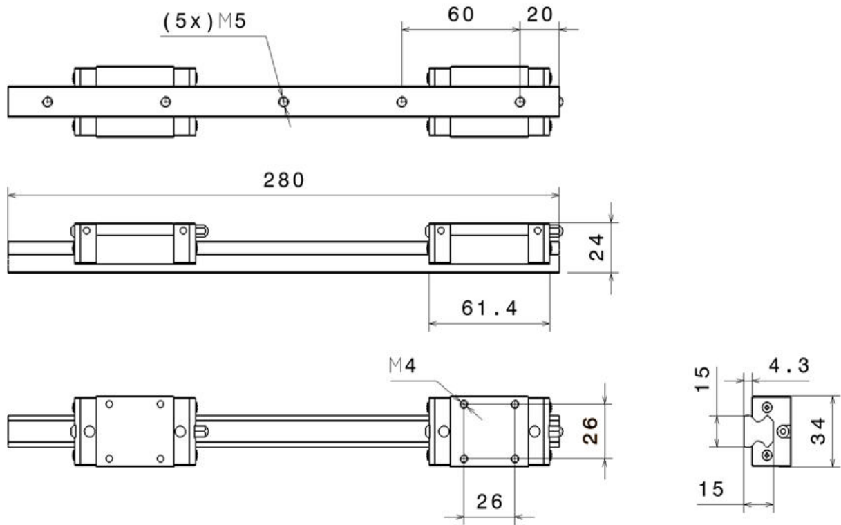
Rys. 2 – Wymagane wymiary gabarytowe [mm]
