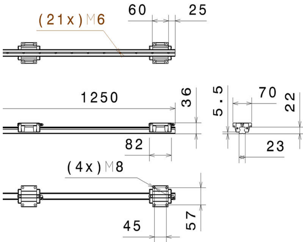
Rys. 1. Wymagane wymiary gabarytowe [mm]
